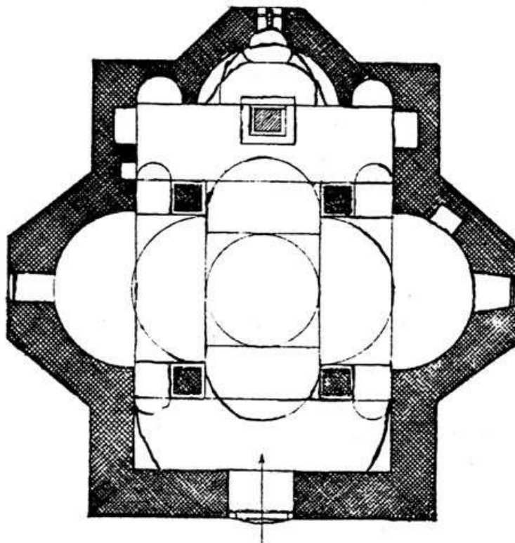
План на храм „Св.Троица”, гр. Разлог
